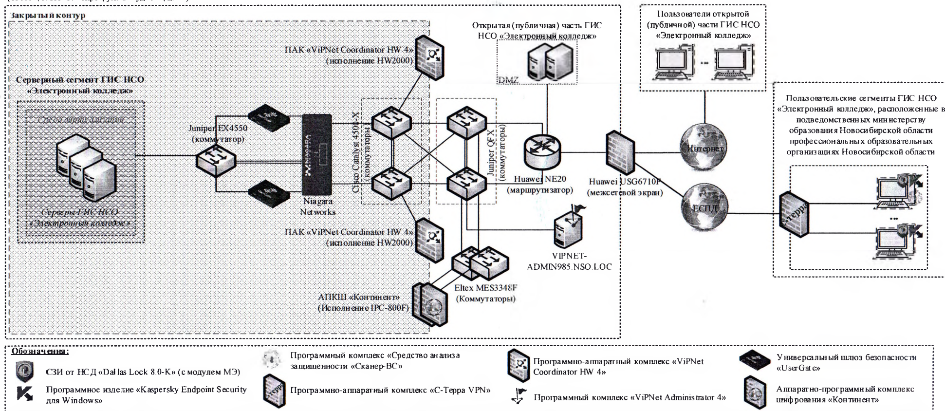
Рисунок 1 - Структурная (топологическая) схема информационных связей ГИС НСО «Электронный колледж»
